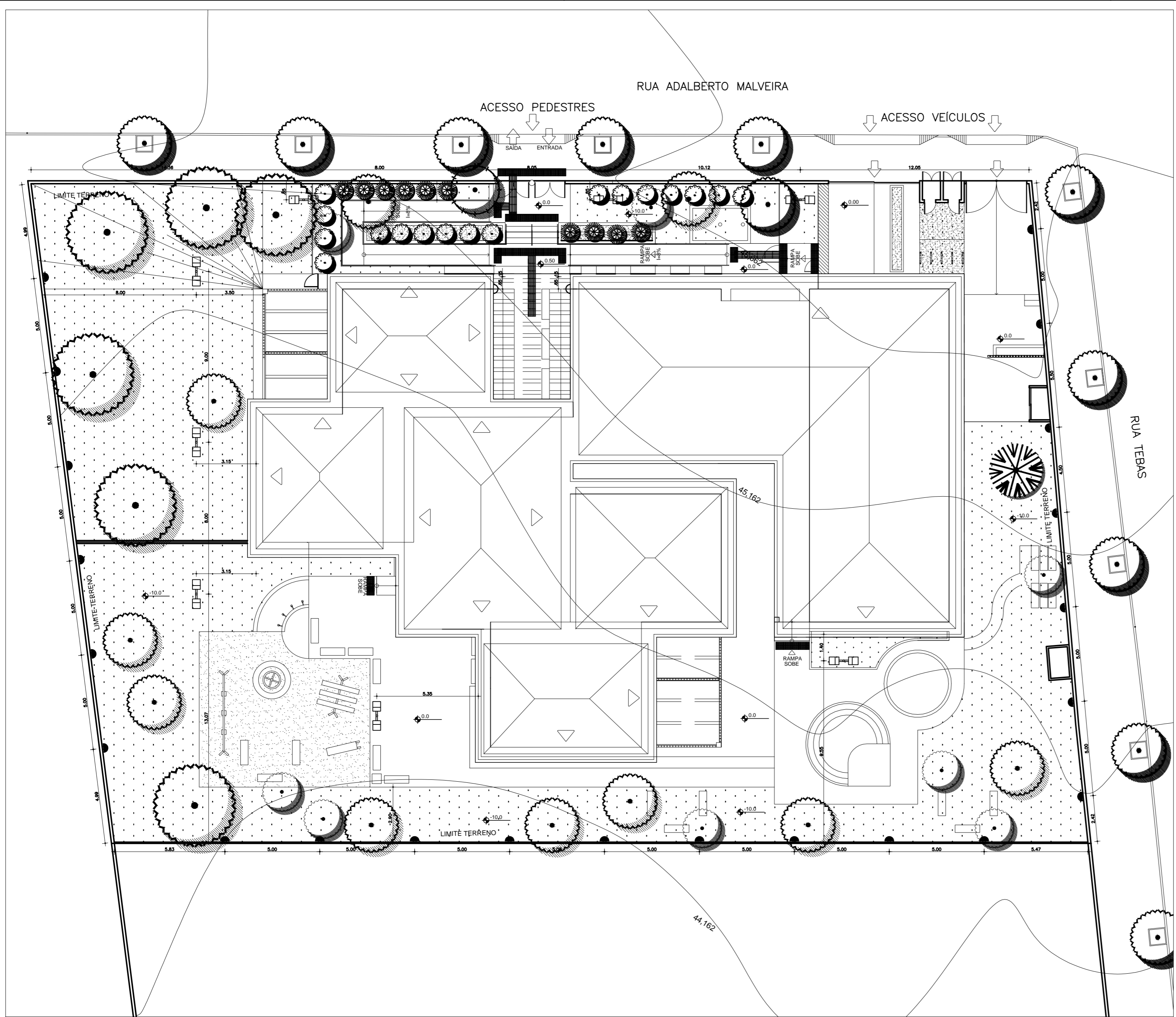
1 PLANTA DE ILUMINAÇÃO ESC.: 1:150
